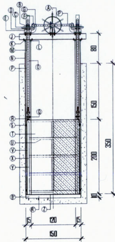
TAMPAK DEPAN/BEKANG
